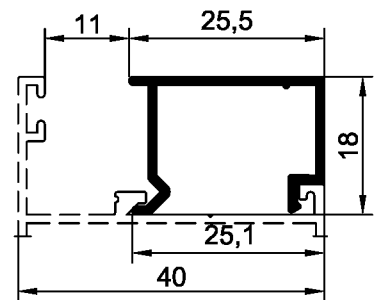
Штапик 25,5
