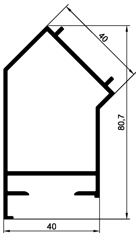
Большой профиль 40x45°
