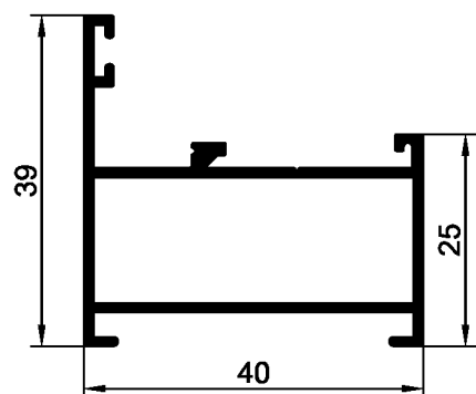
Рамный профиль 25
