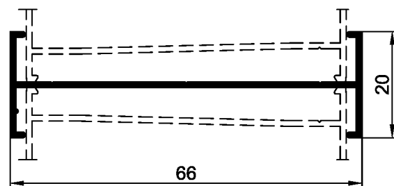
Соединительный профиль 60/60
