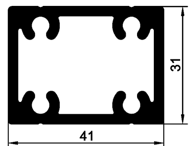
Сухарный профиль
