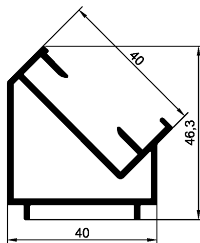
Малый профиль 40x45°
