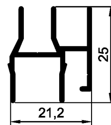
Соединительный профиль
