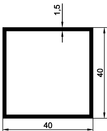
Труба 40x40x1,5
