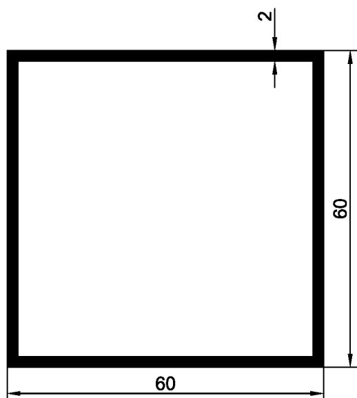
Труба 60x60x2
