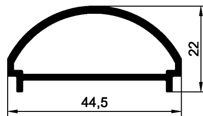
Поворотный профиль
