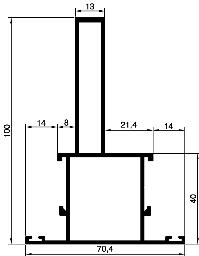
Усиленный Т-образный профиль
