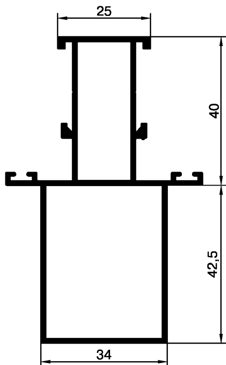
Усиленный профиль 25
