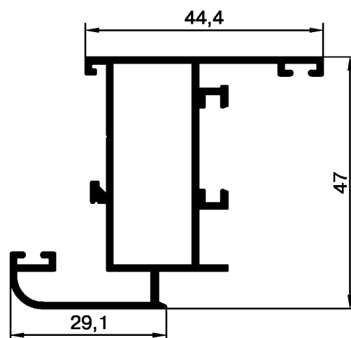
Створочный профиль 44
