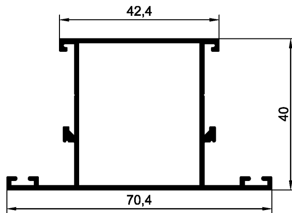
Т-образный профиль 42
