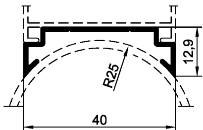
Поворотный профиль 40
