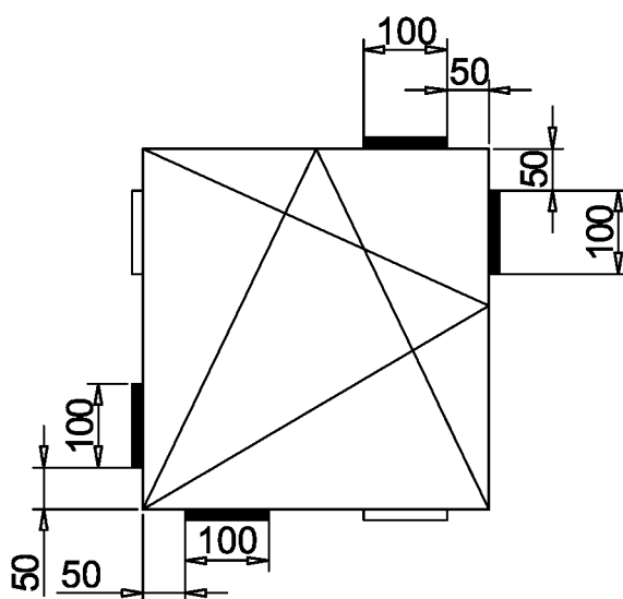
Оконный блок со створкой с поворотно-откидным открыванием
